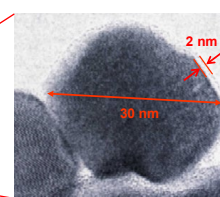
粒子表面に被膜層が観察できる
